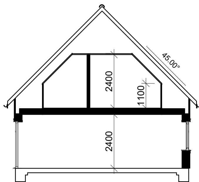
A-A
