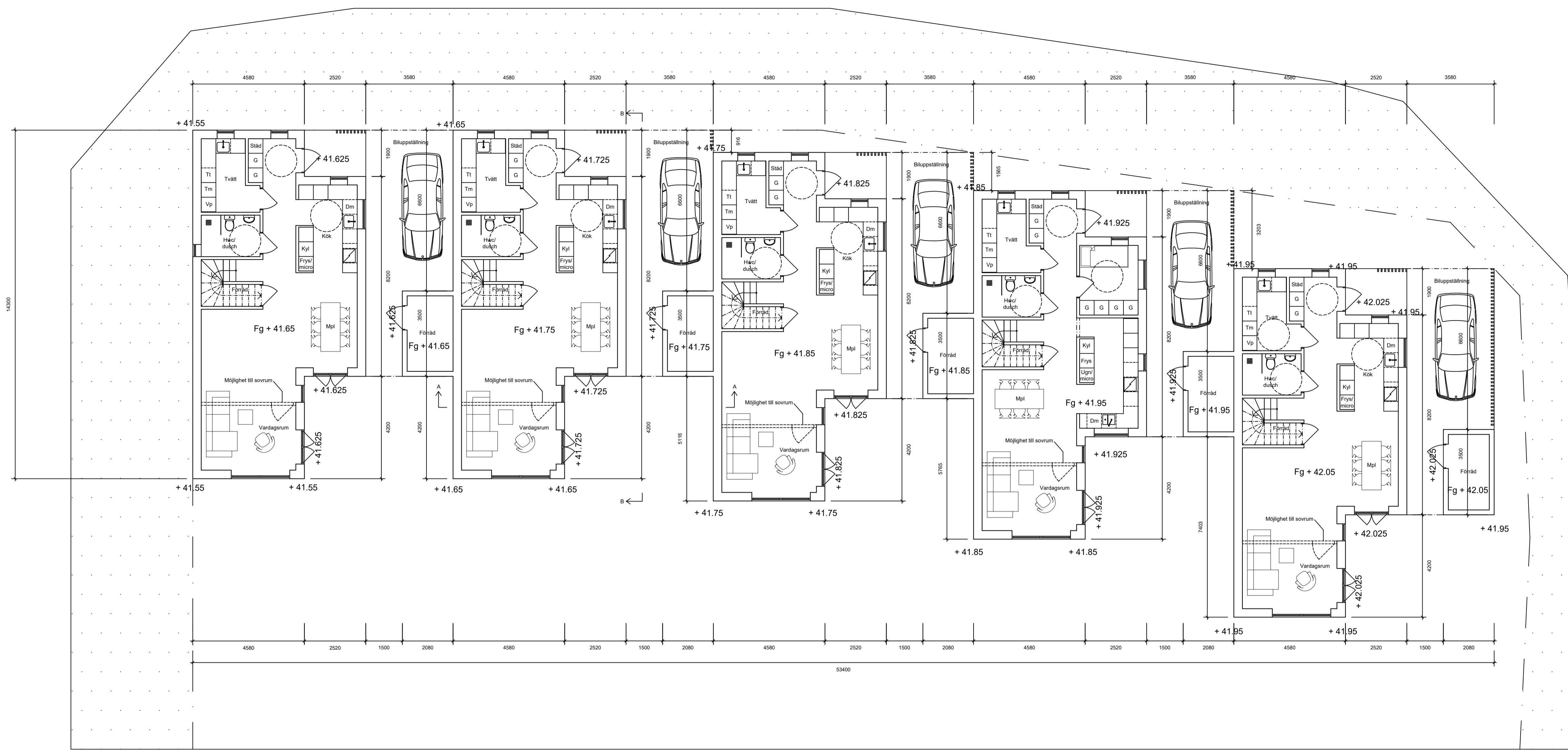
Entréplan, skala 1:100
