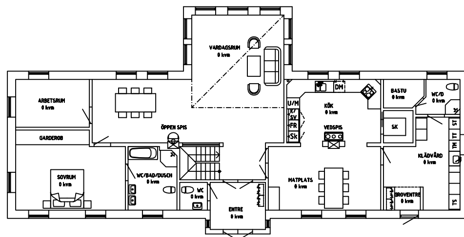
ENTRE PLAN BYGGHADEYTA 225 kvm
