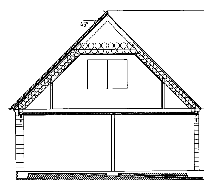
SEKTION D-D
