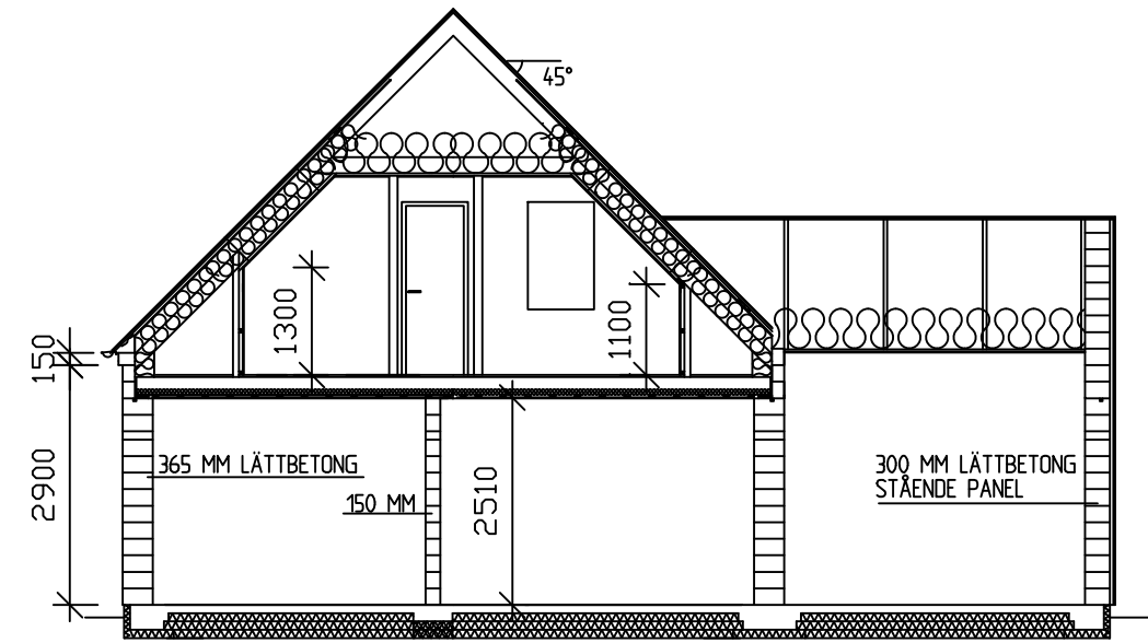
SEKTION A-A
