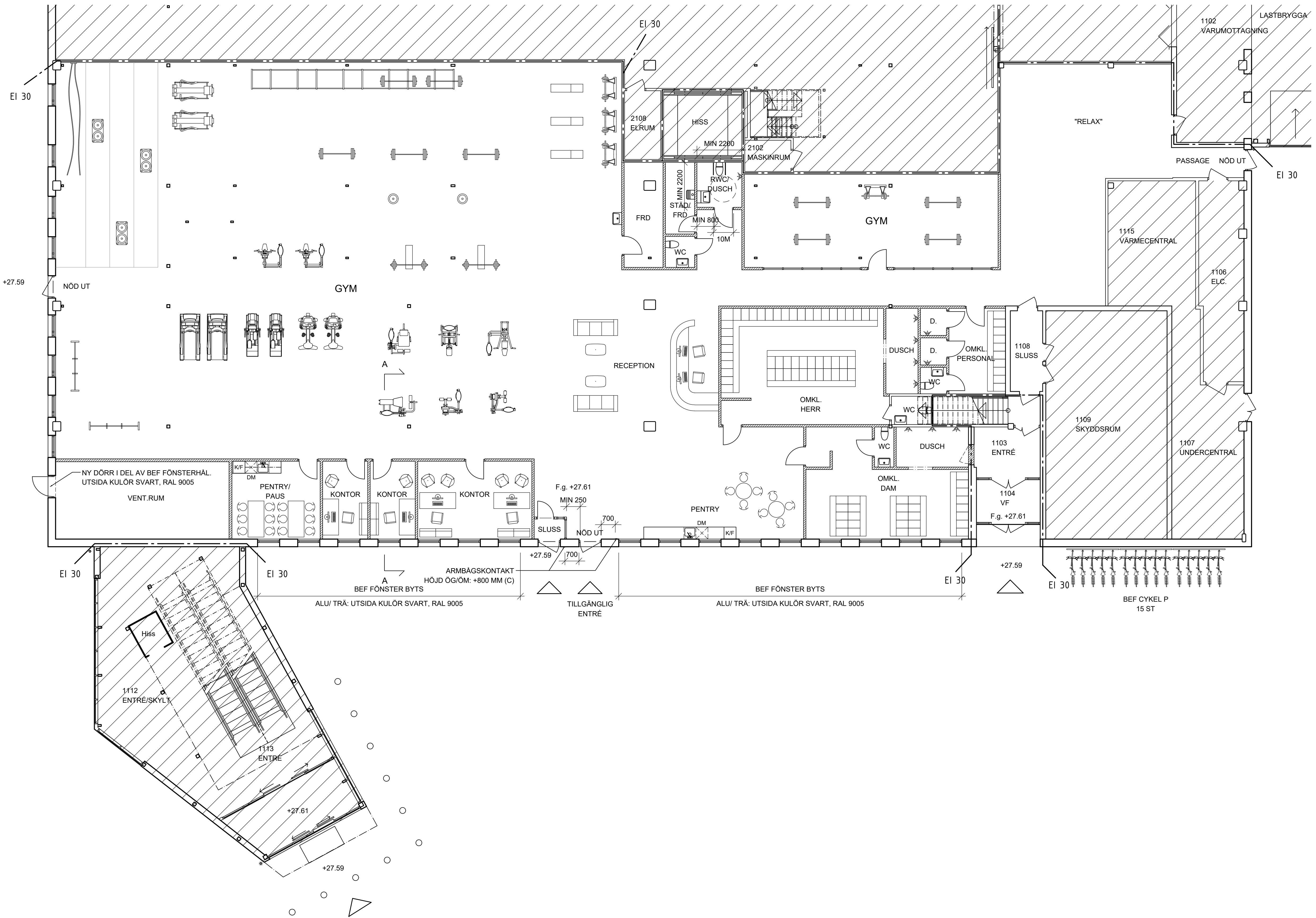
DEL AV PLAN BOTTENVÄNING SKALA 1:100
