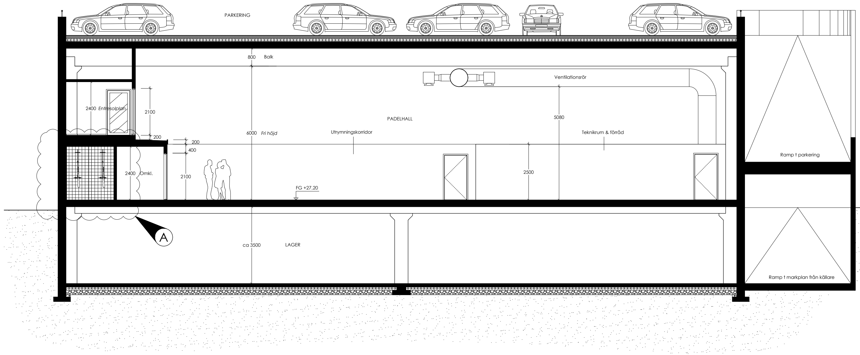
SEKTION A-A Skala 1:100 (A3)
