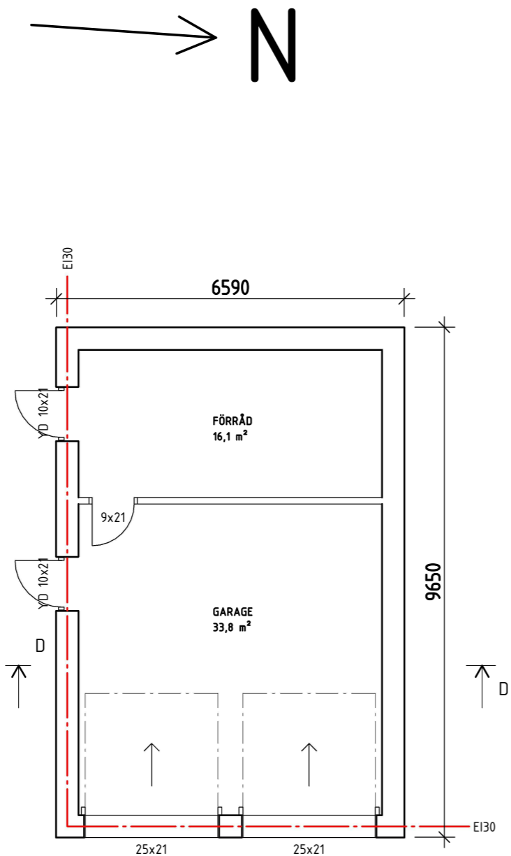
PLAN GARAGE BYGGNADSAREA GARAGE 63,6 m 2
