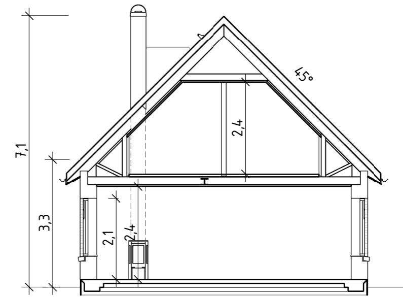
SEKTION C - C
