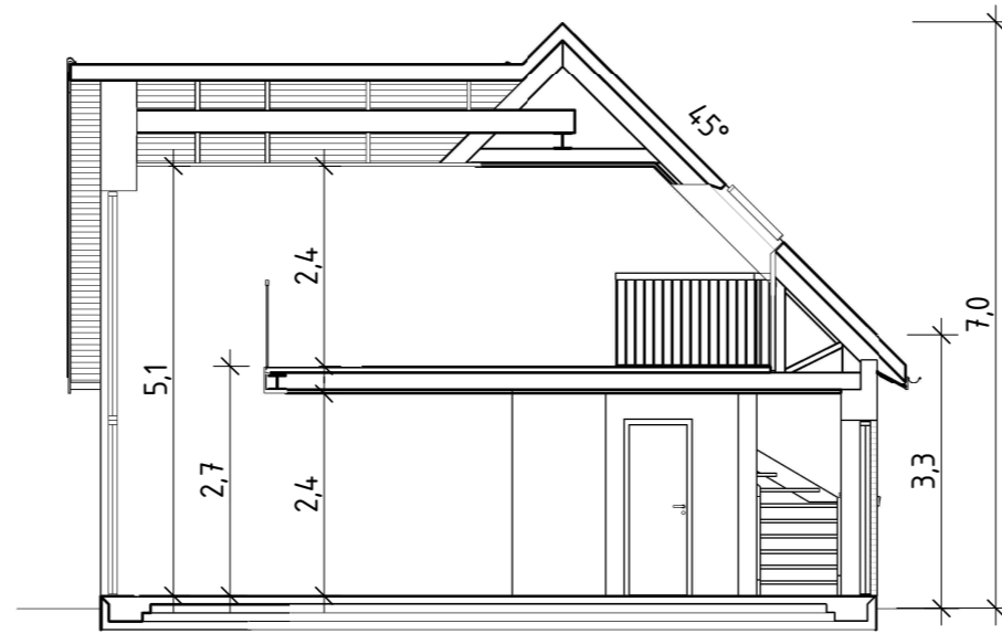
SEKTION B - B
