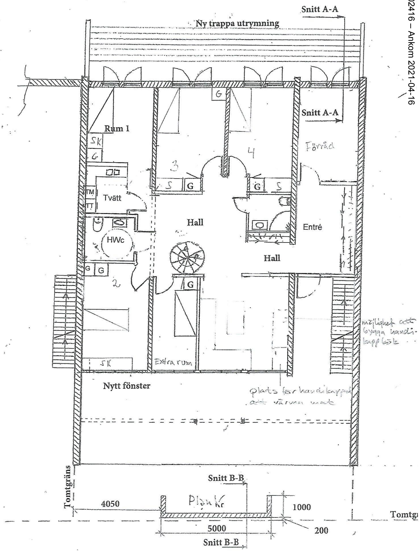
Suterängvåning Skala 1:100
