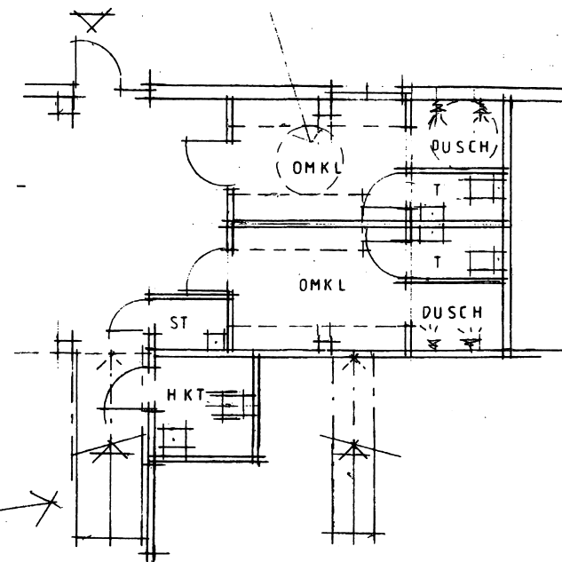
PLAN OMKLÅDN, DEL 1:100
